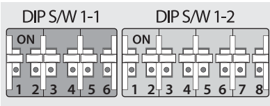
Main PCB Dip 스위치
