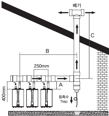
〈FE식 캐스케이드 연통〉
