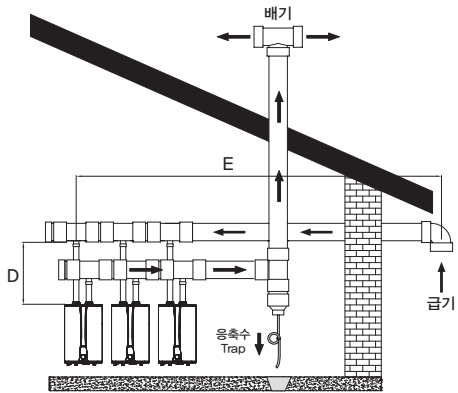
〈FF식 캐스케이드 연통〉
